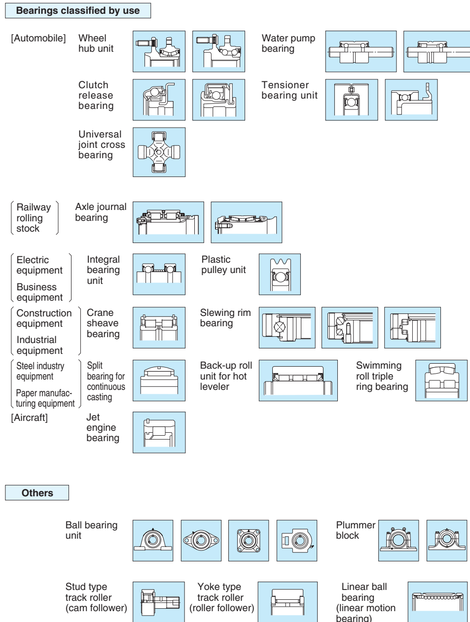
Fig. 1-2(2) Rolling bearings
